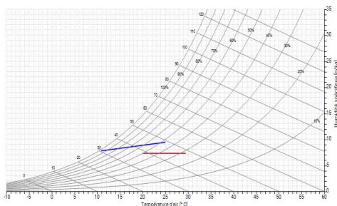
Diagramme Psychrométrique
